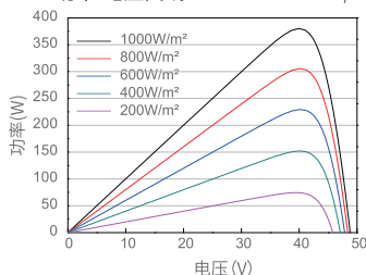
功率-电压曲线 JAM72D09-380/BP
