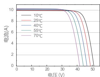
电流-电压曲线 JAM72D09-380/BP
