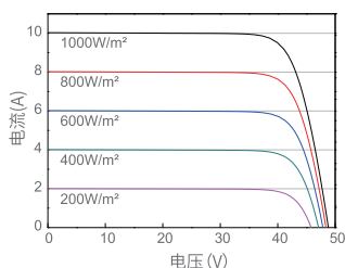
电流-电压曲线 JJAM72D09-380/BP
