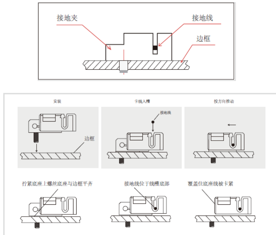
图12 接地夹安装方式
