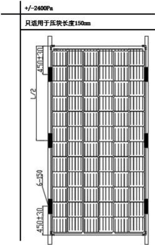
图5-b 72 双面双玻组件安装连接点位置要求（压块）
