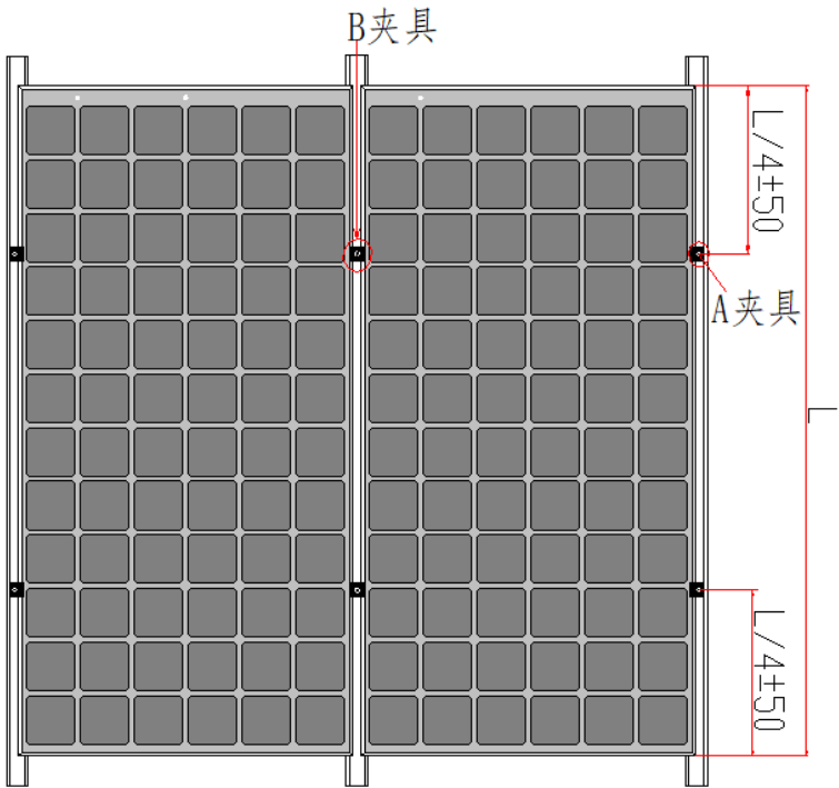
图9 安装细节
