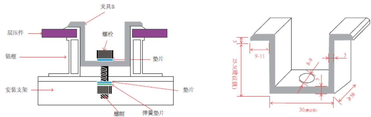
夹具B 中间组件用夹具 图10 安装细节
