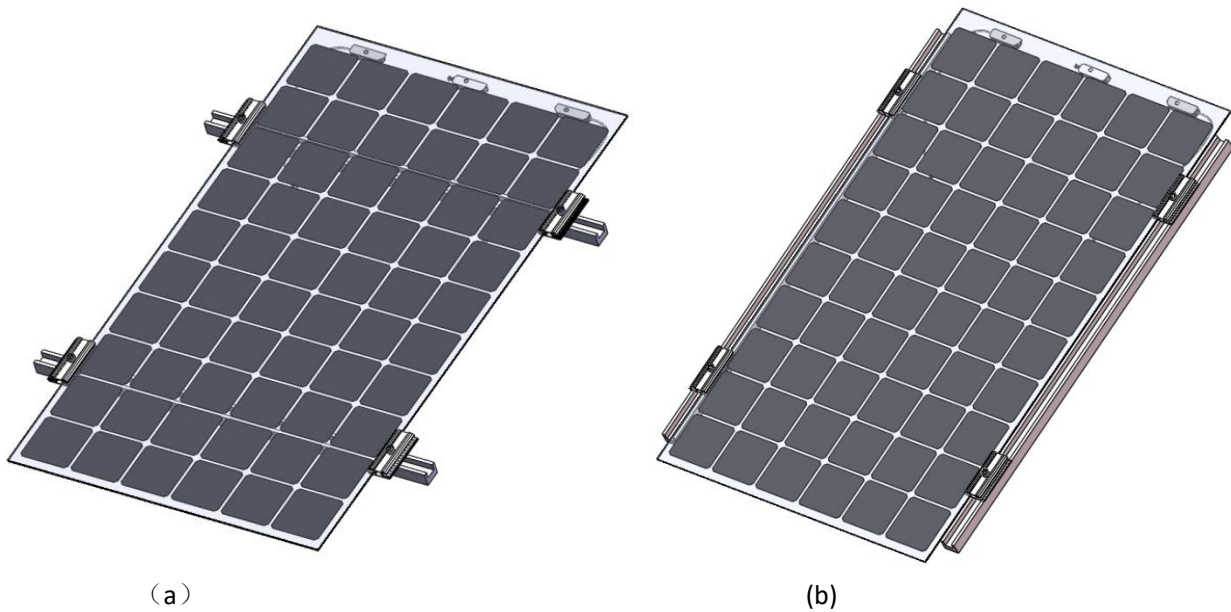
图 2 压块安装图示 (a 图：仅针对无框单面双玻组件；b 图：仅针对无框双面双玻组件)
