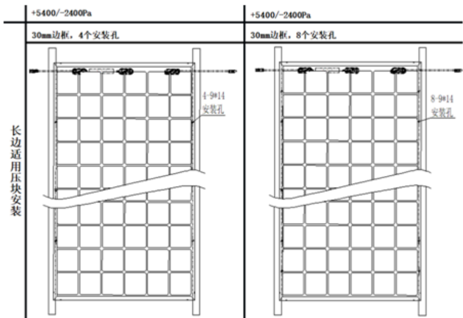
图7 安装位置及对应载荷关系
