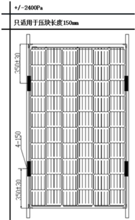
图4-b 60双面双玻组件安装连接点位置要求（压块）
