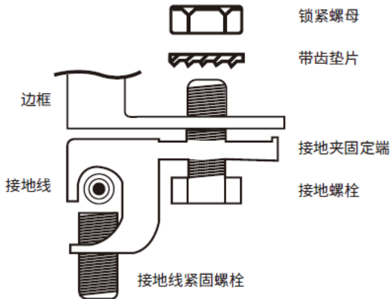
图 13 安装方式
